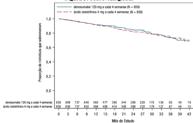
Figura 3. Sobrevida global
